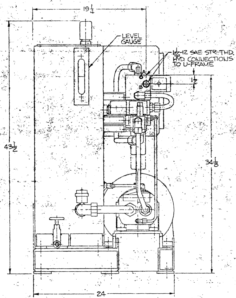
ELEVATION
