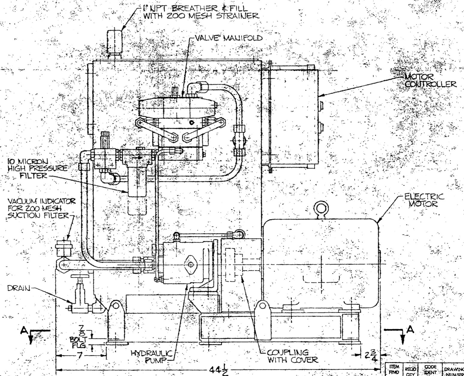
ELEVATION
